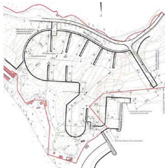
Slika 5. Osnovni prostorni parametri pomorsko građevinskih objekata luke Kuje
